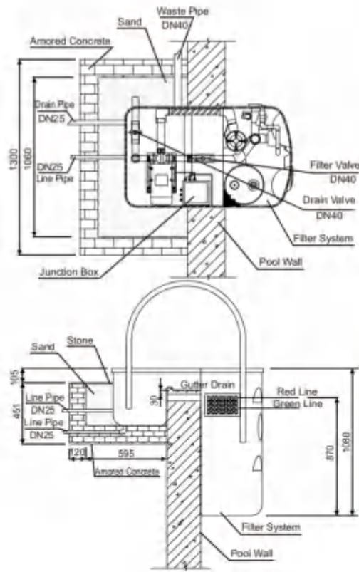
PM-GL25Y
