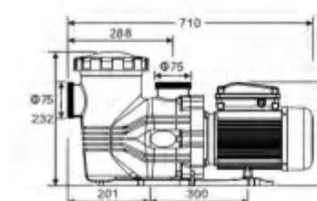
WL-BDP400
