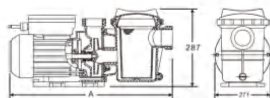
WL-STP150-WL-STP300
