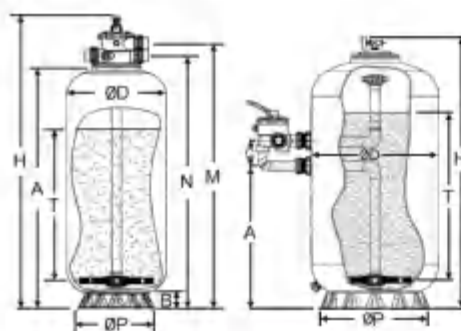
WL-DDG13400-WL-DDG15700
