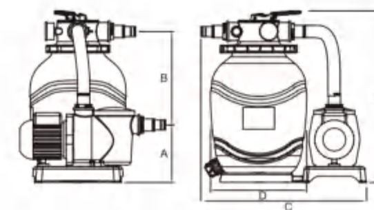
RDG300K
