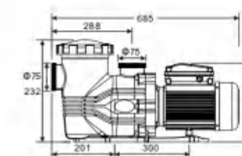
WL-BDP200
