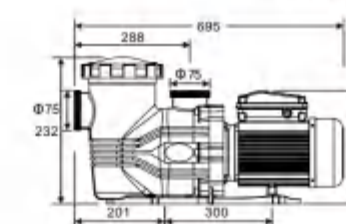
WL-BDP300
